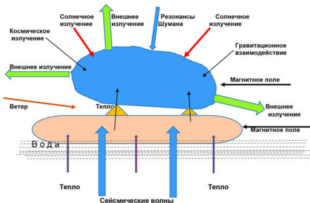
Рис. 47. Факторы, влияющие на сейды
