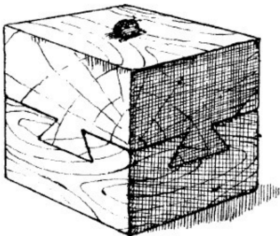
Рис. 2.20. Хитроумное соединение в собранном виде
