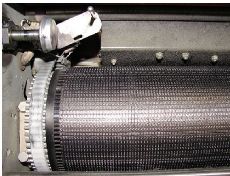
Рис. 3.8. Барабанный принтер 26
