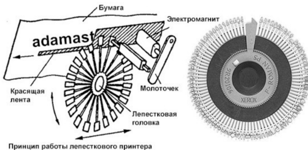
Рис. 3.9. Лепестковый принтер 27
