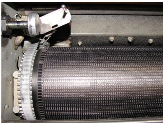
Рис. 3.8. Барабанный принтер 26
