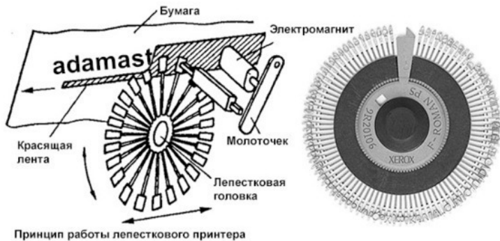
Рис. 3.9. Лепестковый принтер 27
