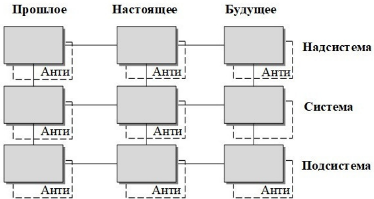
Рис. 2.12. Системный оператор
