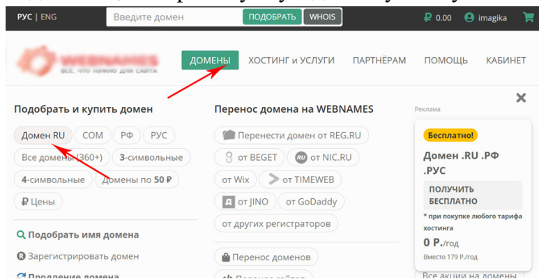
Рис. 10. Регистрация домена
