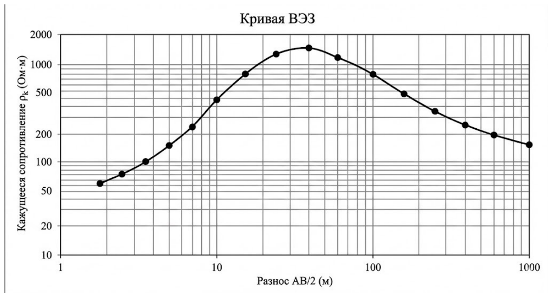
Кривая ВЭЗ
