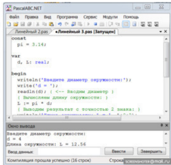
Рис.15. Программа на языке Паскаль и ее реализация в системе программирования
