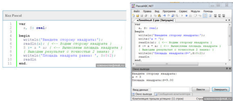
Рис.12. Программа на языке Паскаль и ее реализация в системе программирования Pascal ABC.NET .
