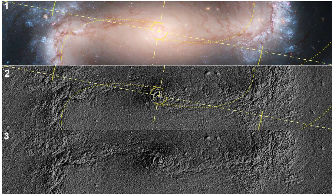
Рис. 8. Сравнение смоделированной линии фронта частиц и фотографии ядра галактики NGC 1300. Источник – ESA/Hubble ( https://cdn.esahubble.org/archives/images/large/opo0501a.jpg ). Исходная фотография повернута на 20^\circ и из нее выбран горизонтальный фрагмент, захватывающий ядро галактики. Кадр 1 – на фотографию наложена смоделированная спираль при скорости частиц v=0.763c . Кадр 2 – та же спираль наложена на 3D-рельеф, сгенерированный программой на основе исходной фотографии. Кадр 3 – только 3D-рельеф
