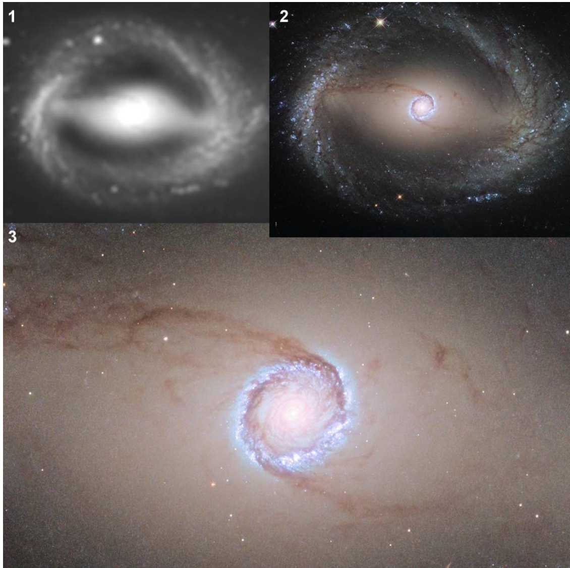
Рис. 2. Галактика NGC 1512. Источник – ESA/Hubble ( https://cdn.esahubble.org/archives/images/large/heic1712a.jpg ). Используется только левая половина снимка с собственно галактикой NGC 1512. Кадр 1 – ухудшенное исходное изображение. Кадр 2 – уменьшенное исходное изображение. Кадр 3 – центральная часть галактики из того же исходного изображения.
