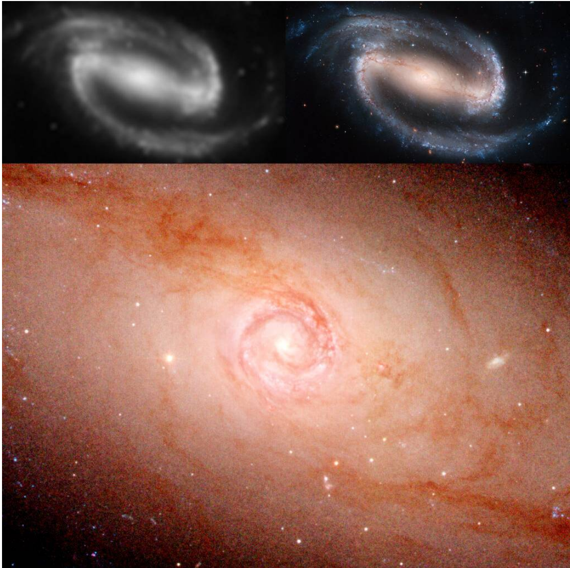
Рис. 1. Галактика NGC 1300. Источник – ESA/Hubble ( https://cdn.esahubble.org/archives/images/large/opo0501a.jpg ). Кадр 1 – получен из оригинального (кадр 2) с использованием графических фильтров (обесцвечивание, уменьшение размера, размытие), чтобы продемонстрировать то, как выглядели снимки этой галактики полсотни лет назад. Кадр 2 – уменьшенное изображение ESA/Hubble. Кадр 3 – центральная часть исходного изображения ESA/Hubble (снижена яркость, поднята контрастность).
