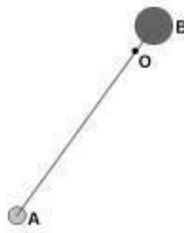
Рис. 11. Квазар J1601+3102. Схема расположения ЧД (точка O), северного (B) и южного (A) выбросов радио-джета. Выброс B значительно ближе к источнику и намного «ярче».
