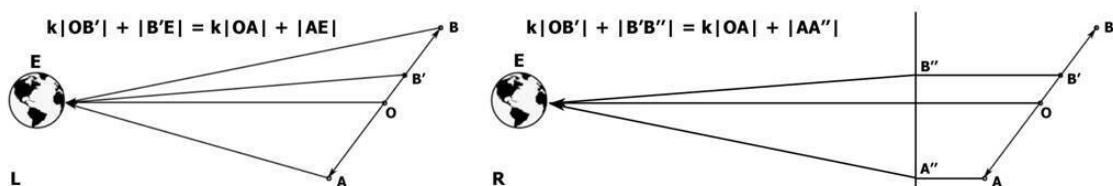
Рис. 10. Постановка задачи об учете задержки сигнала от объектов при движении их из точки O в противоположных направлениях A и B со скоростями v=kc , где 0 < k \leq 1 . Слева – точная постановка задачи, справа – упрощенная. Рисунок автора.
