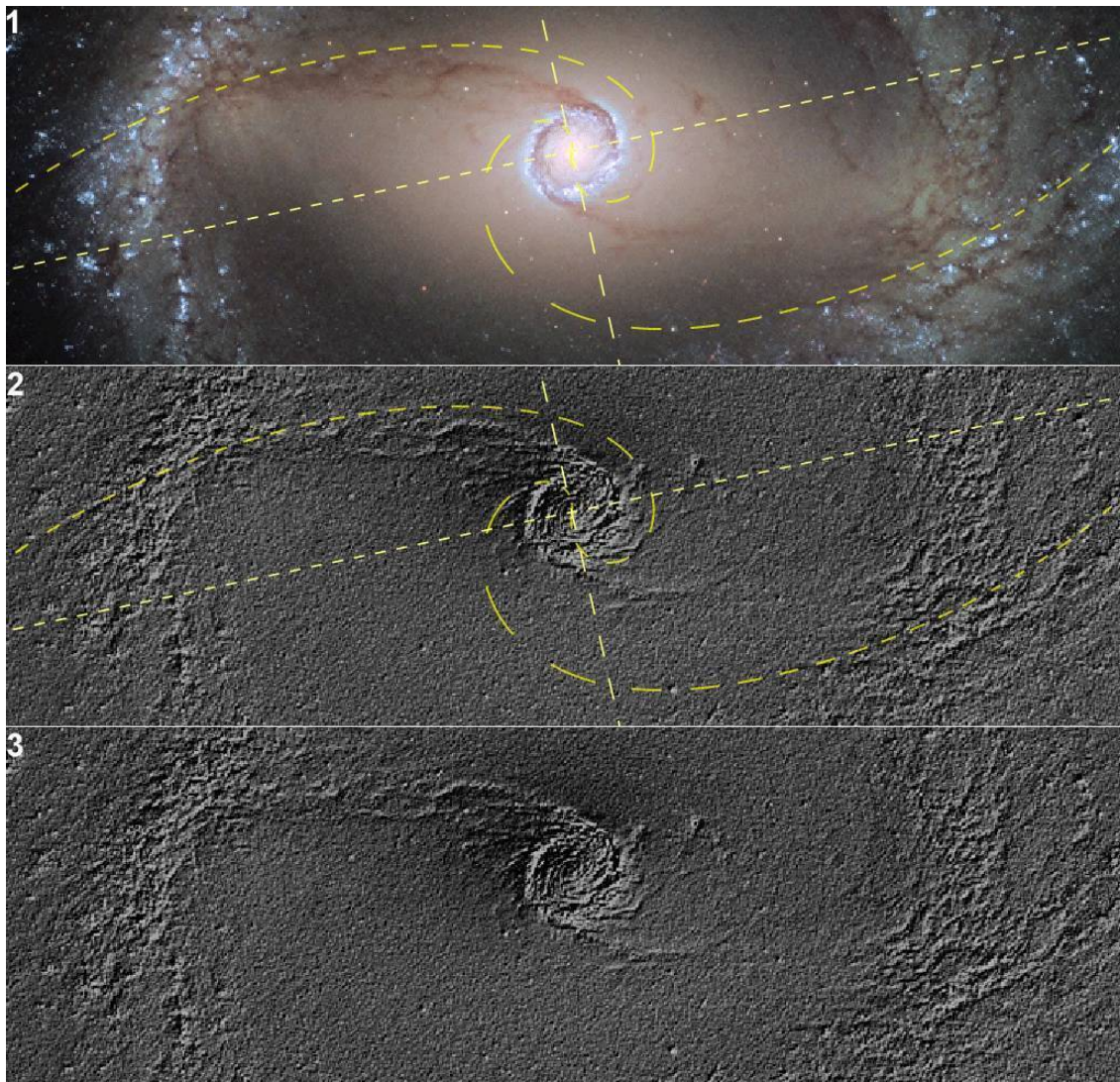
Рис. 7. Сравнение смоделированной линии фронта частиц и реальной фотографии ядра галактики NGC 1512. Источник – ESA/Hubble ( https://cdn.esahubble.org/archives/images/screen/ )
