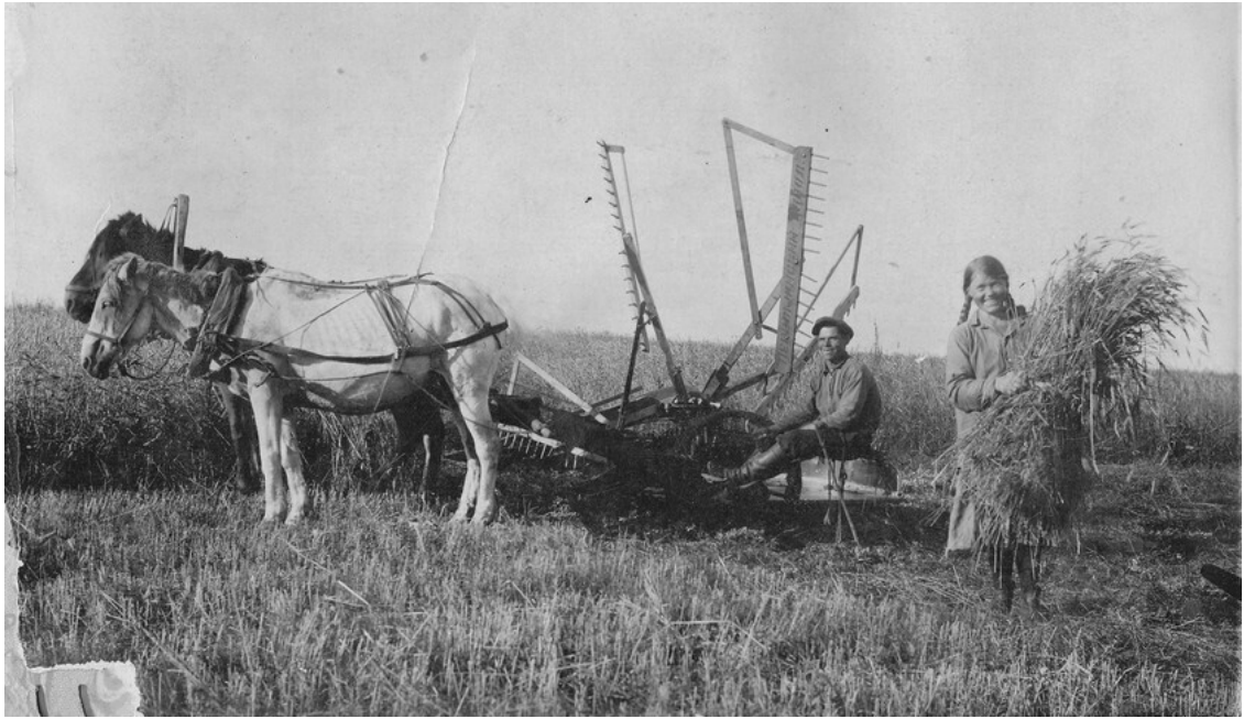
Рис. 18. Конная жатка (лобогрейка)
