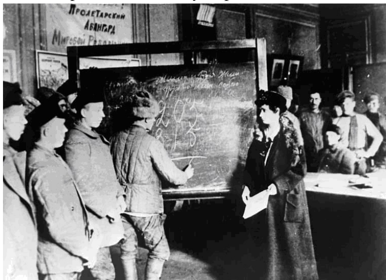
Рис. 35. Обучение счёту
