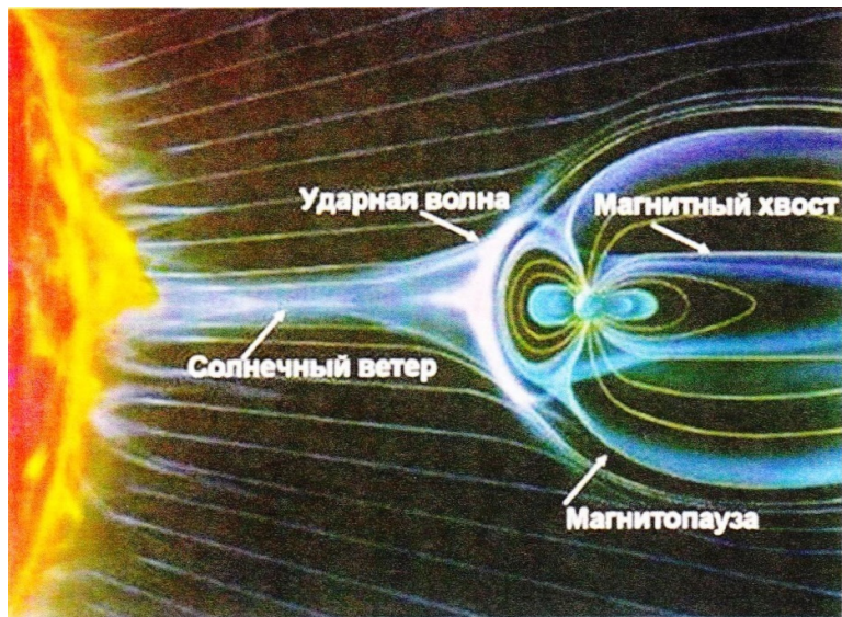
Рис. 5. Магнитосфера о-т Земли
