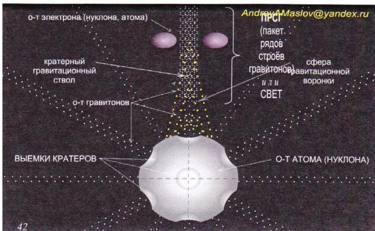
Рис. 4. Процесс образования лучей света (ПРСГ) — 2 этап
