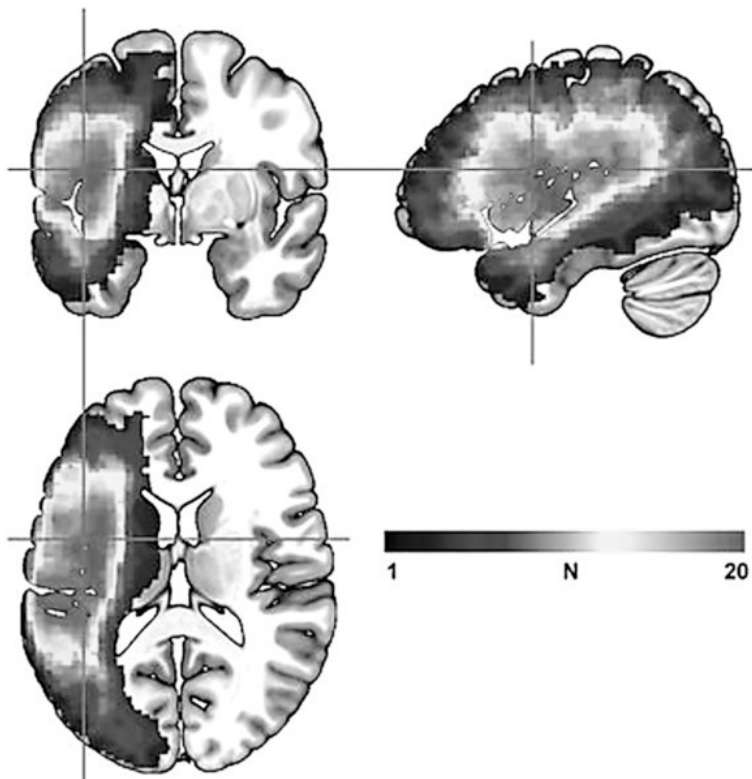
Рис. 3. Карты наложения очагов поражения для для 20 пациентов с эфферентной моторной афазией. Перекрестия обозначают воксель, где наблюдалось наибольшее перекрытие очагов поражения [Fridriksson J et al., 2015]
