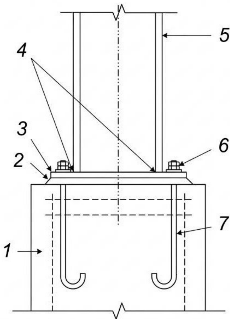
1- Бетонный фундамент; 2 — Раствор; 3 — Опорная плита; 4 — Стыковой шов; 5 — Стальная колонна; 6 — Двойные контргайки и шайба; 7 — Анкерный болт. Рисунок 4 — Крепление колонн к фундаменту
