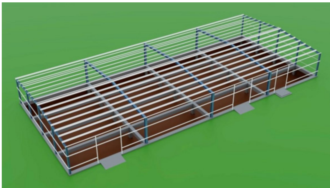
Рисунок 3 — Каркас здания мини-завода
