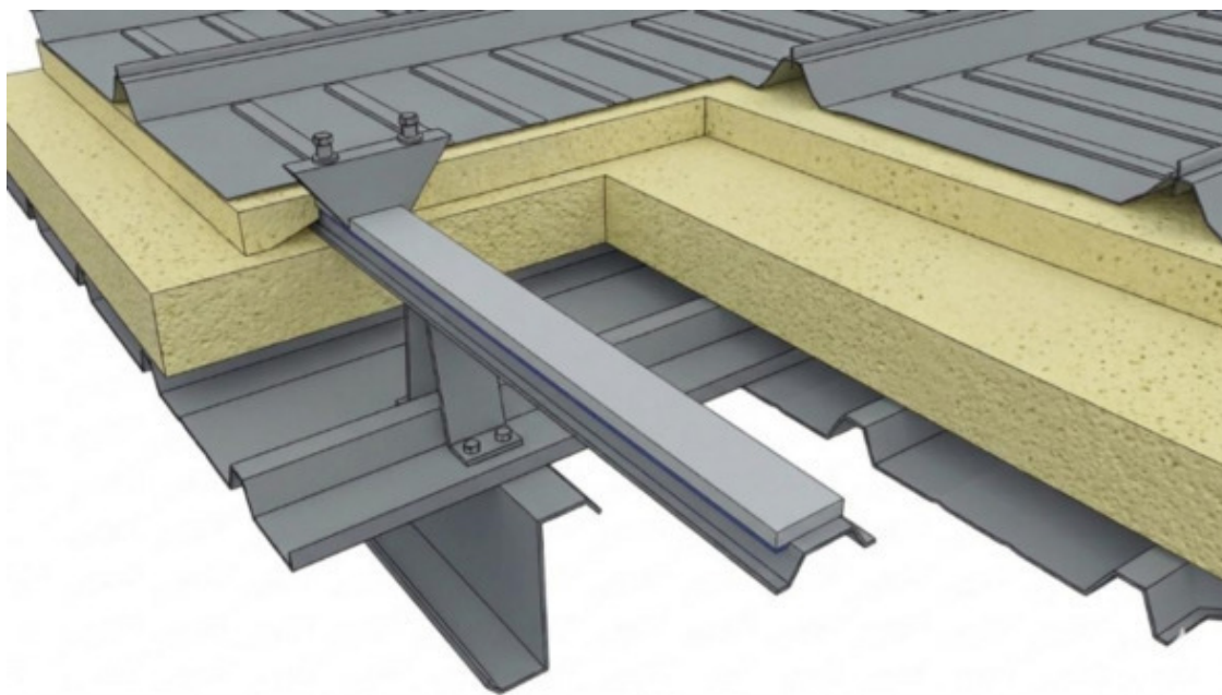
Рисунок 5 — Двухслойная стальная фальцевая кровельная система
