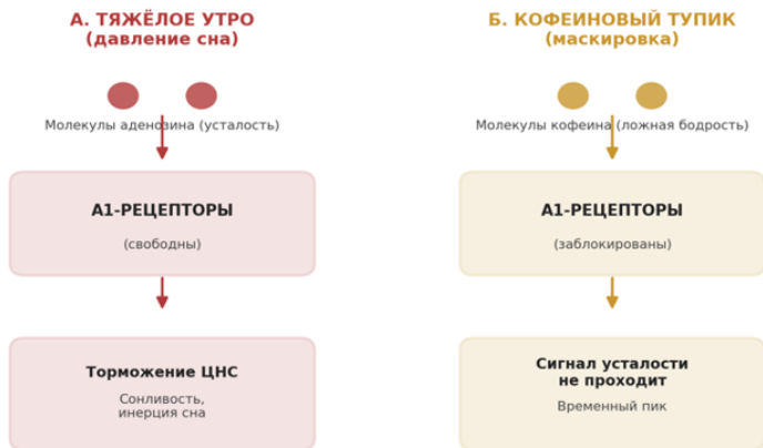
Рисунок 7.3. Физиология инерции сна (Аденозин vs Кофеин)
