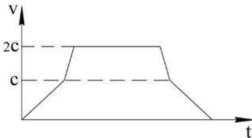
Рисунок 1 Полет со скоростью 2c
