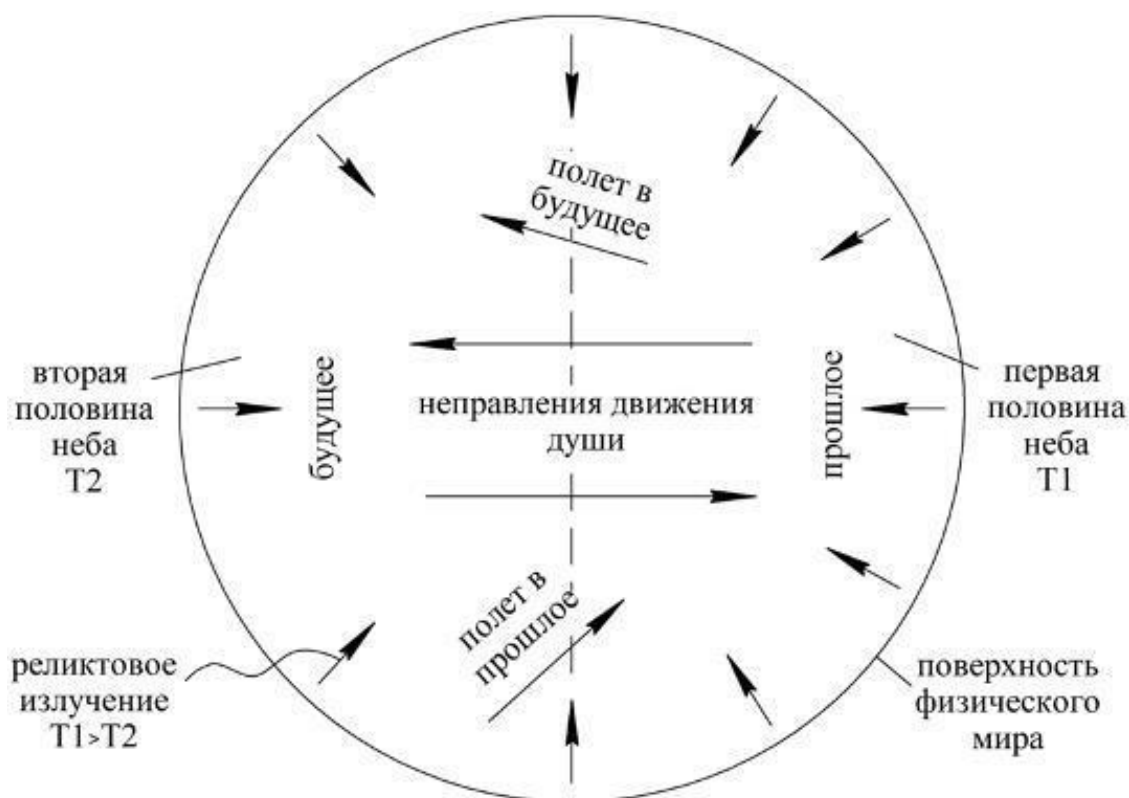
Рисунок 3 Полет во времени и в пространстве
