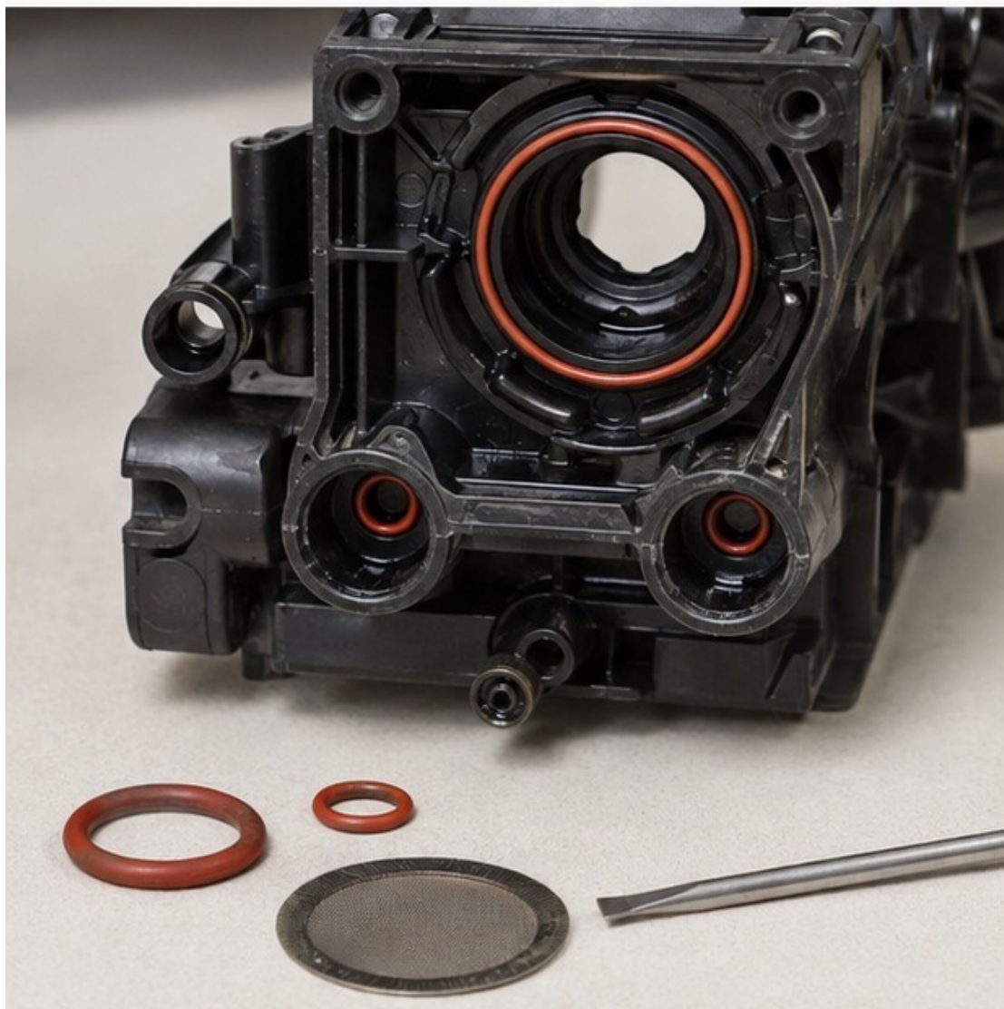
Уплотнения гидравлического блока кофемашины.
