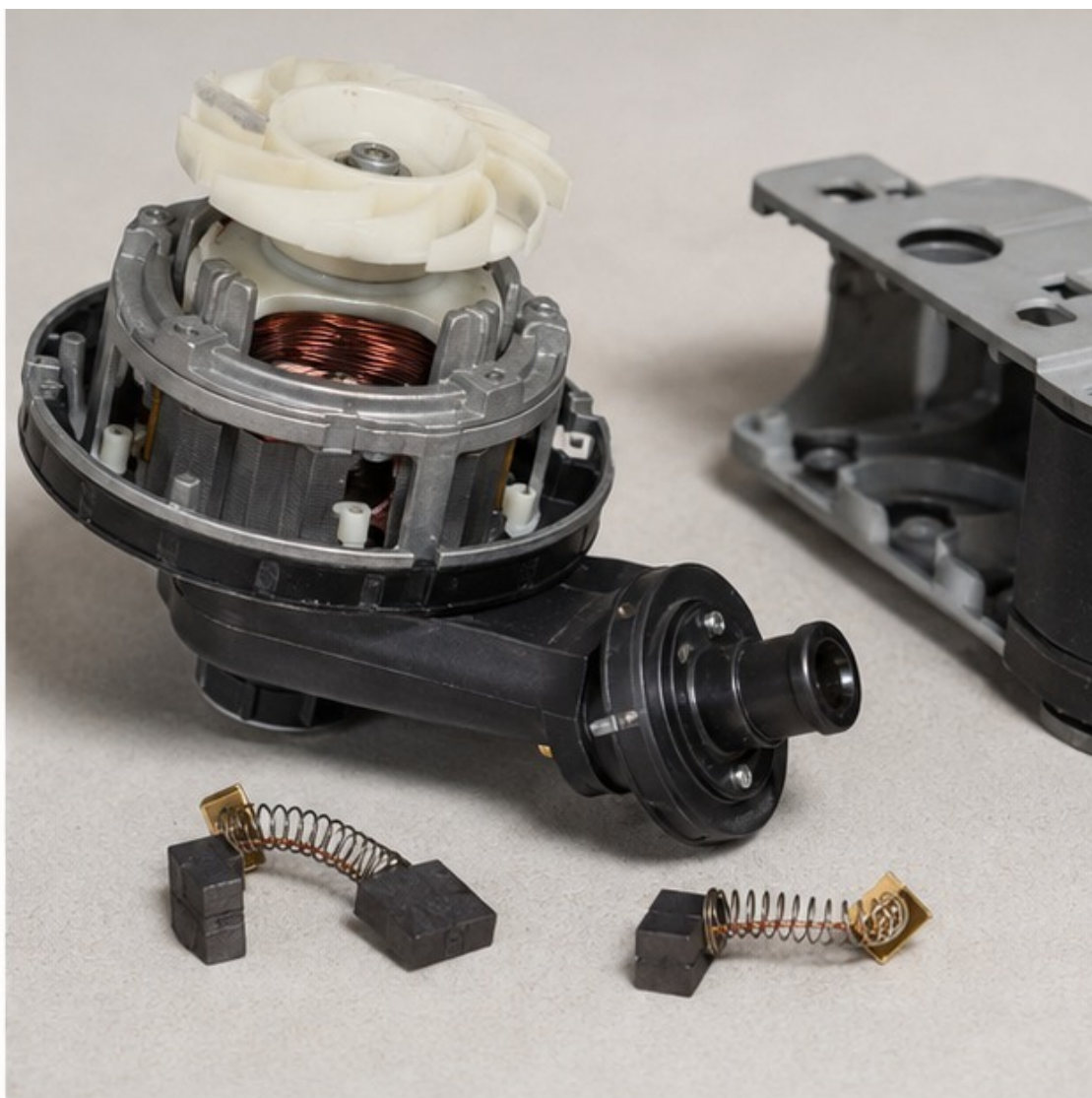
Двигатель и угольные щётки кухонного прибора.
