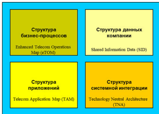
Рис.4.7. Методология NGOSS
