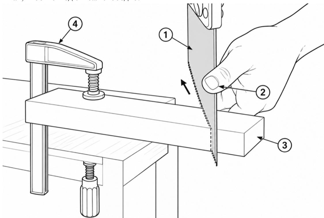
Рисунок 4.4. Начало реза. Большой палец направляет полотно, полотно вертикально, отход свисает за опорой.
