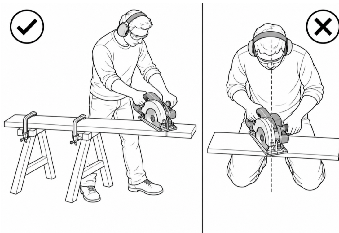
Рисунок 3.1. Слева правильно: тело сбоку от линии диска, доска на двух опорах у линии реза, отрезок свисает. Справа неправильно: тело за пилой, доска на коленях.
