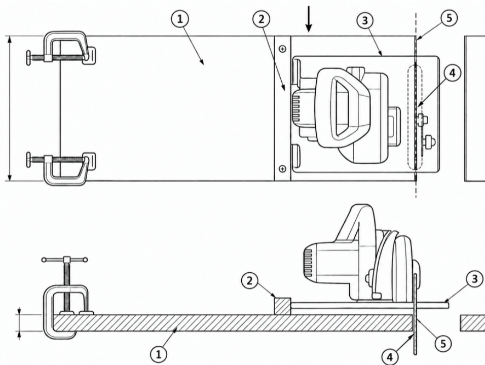
Рисунок 4.5. Основание из фанеры, упор из заводской кромки, первый проход подрезает основание по диску. Размеры в миллиметрах.
