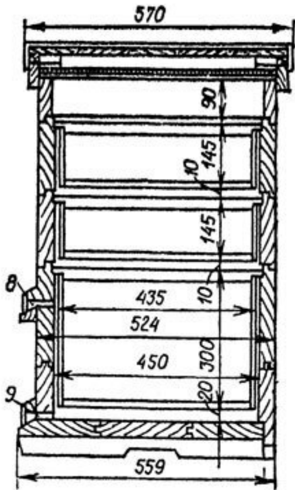
Устройство двенадцатрамочного улья с двумя
