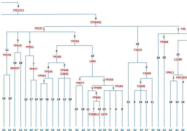
Рис. 31. Диаграмма снипов субклада CTS3402. Показаны три основные нисходящие ветви со снипами YP237, Y33 и Y2613 (1, 1, и 10 снипов от родительского субклада CTS3402), и далее происходит дробление на нижеследующие ветви. Числа внизу: общее число снипов от R1a>Z280 (Рис. 4) [5. Клёсов]
