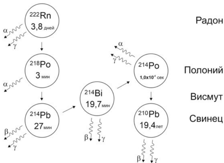
Рис. 1. Схема радиоактивного распада радона и его ДПР.
