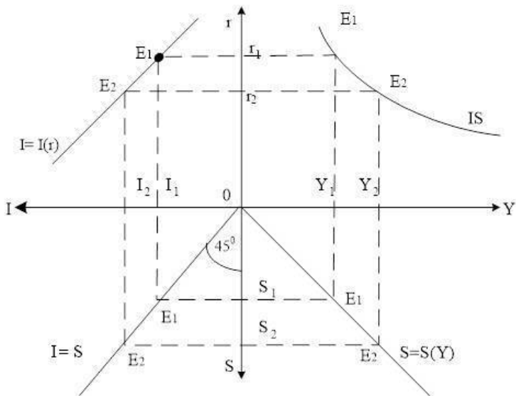
Рис.1 Построение графика IS
